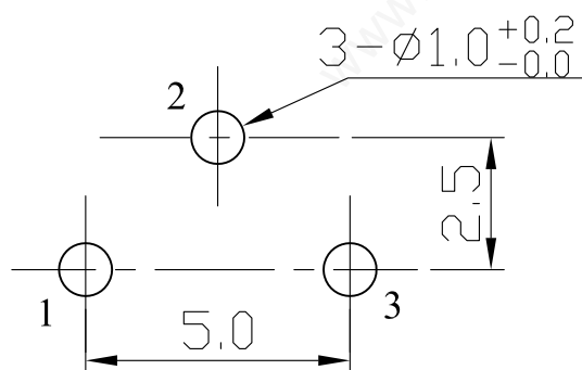
安裝孔位置圖 Mounting Hole
